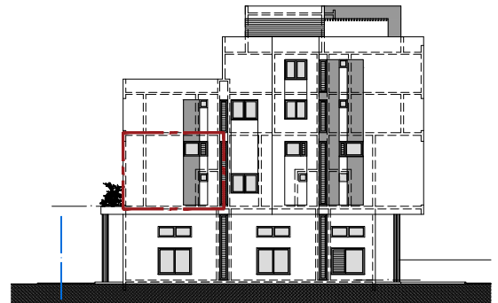
ELEVATION 2
